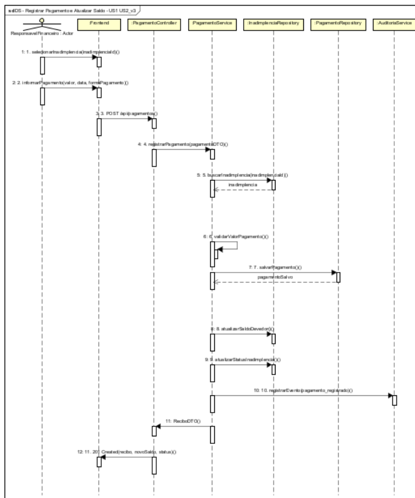
Figura 12 — Diagrama de Sequência: Registrar Pagamento e Atualizar Saldo — US1 e US2.
