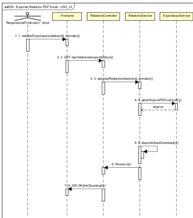
Figura 15 — Diagrama de Sequência: Exportar Relatório PDF/Excel — US5.
