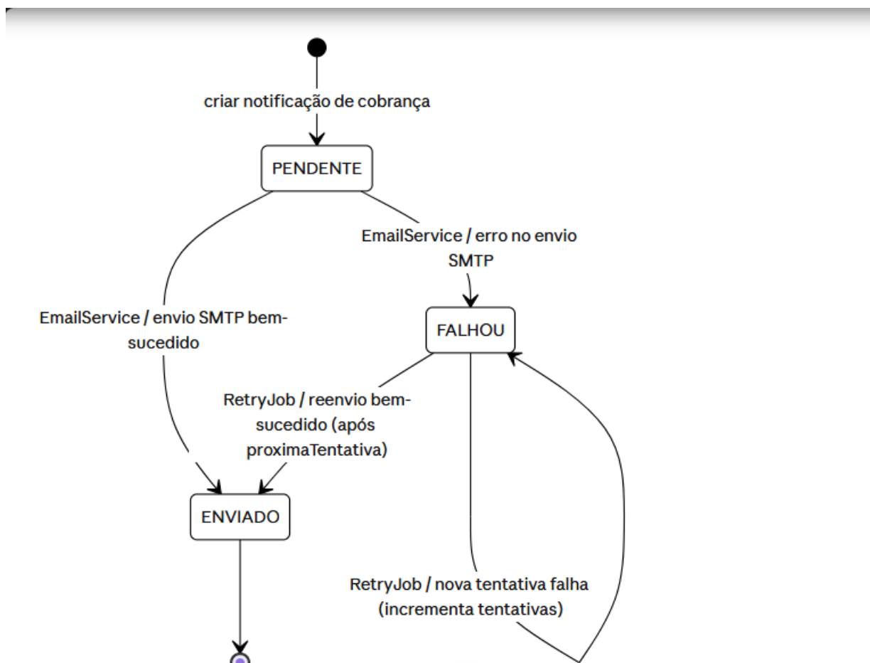
Figura 33 — Diagrama de Estado.
