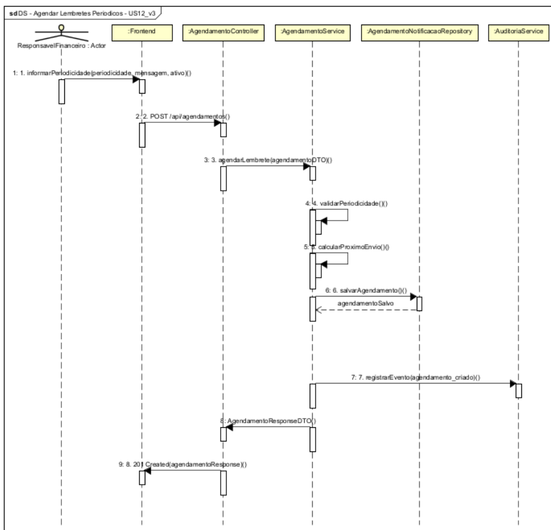
Figura 19 — Diagrama de Sequência: Agendar Lembretes Periódicos — US12.
