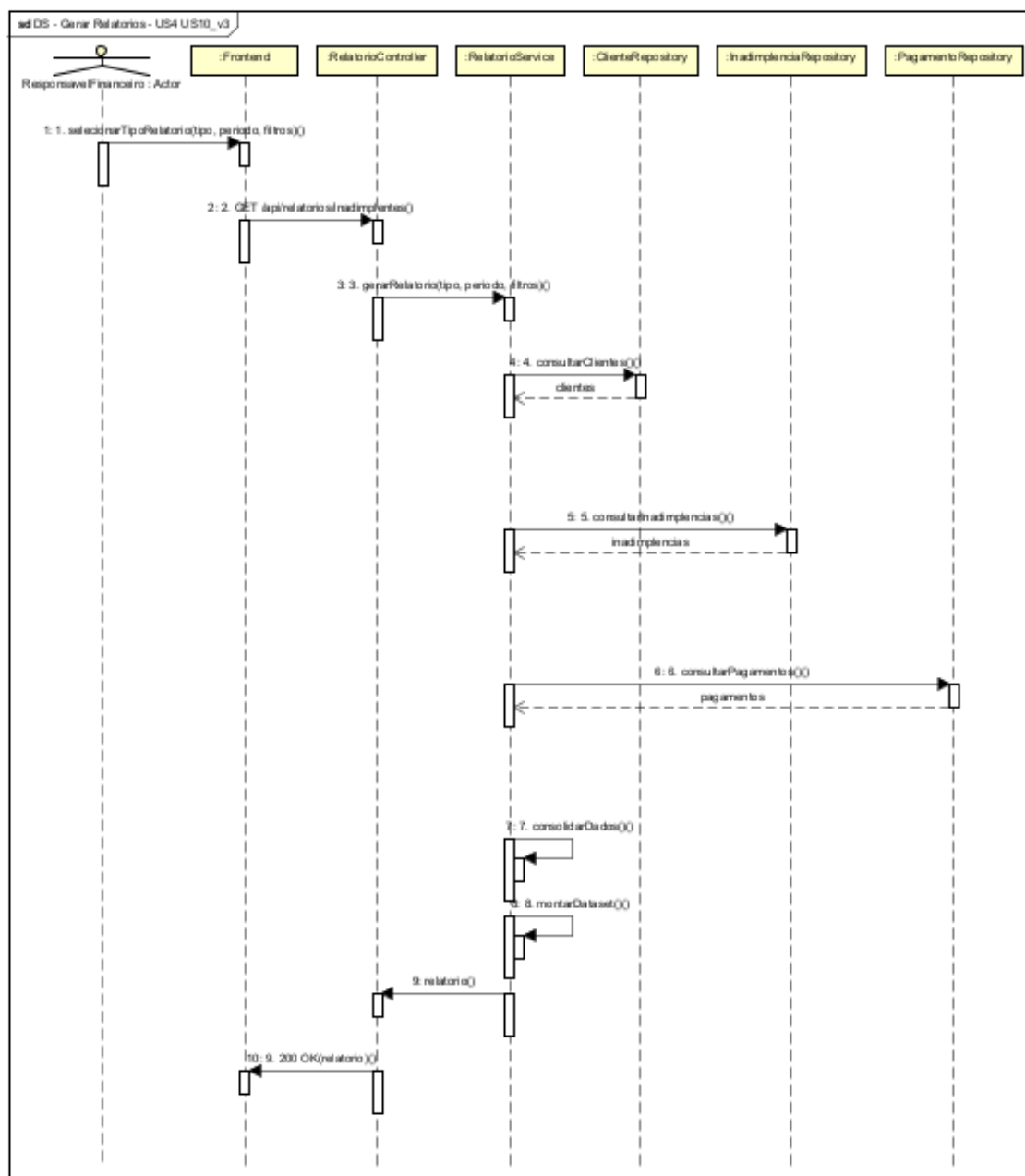
Figura 14 — Diagrama de Sequência: Gerar Relatórios — US4 e US10.
