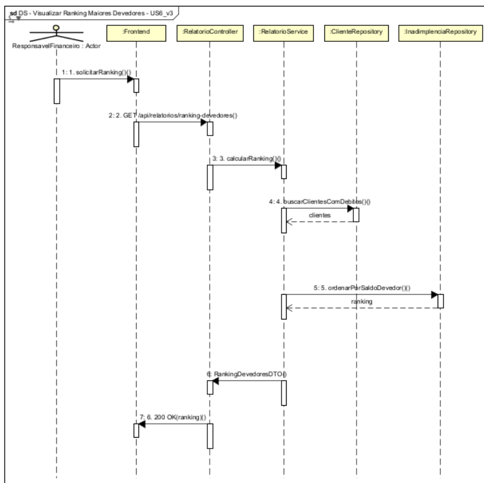
Figura 16 — Diagrama de Sequência: Visualizar Ranking de Maiores Devedores — US6.
