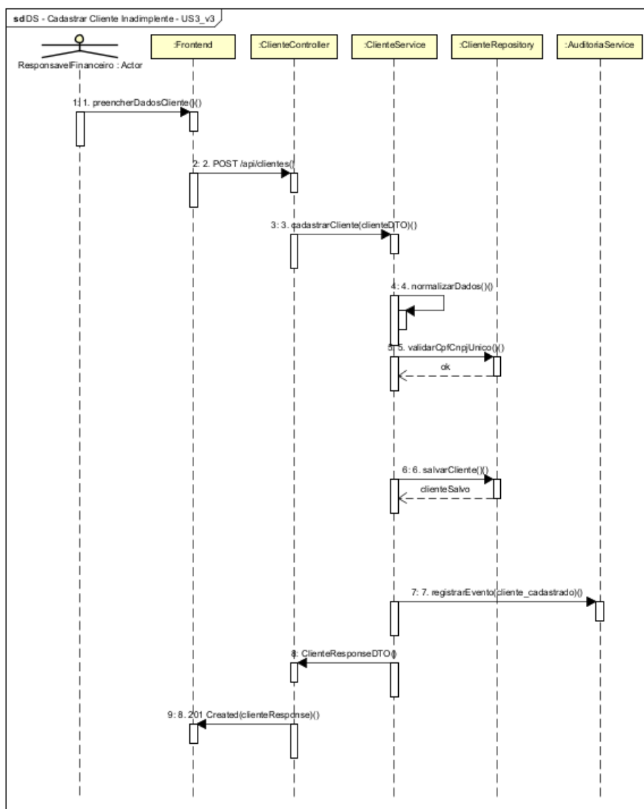
Figura 9 — Diagrama de Sequência: Cadastrar Cliente Inadimplente — US3.
