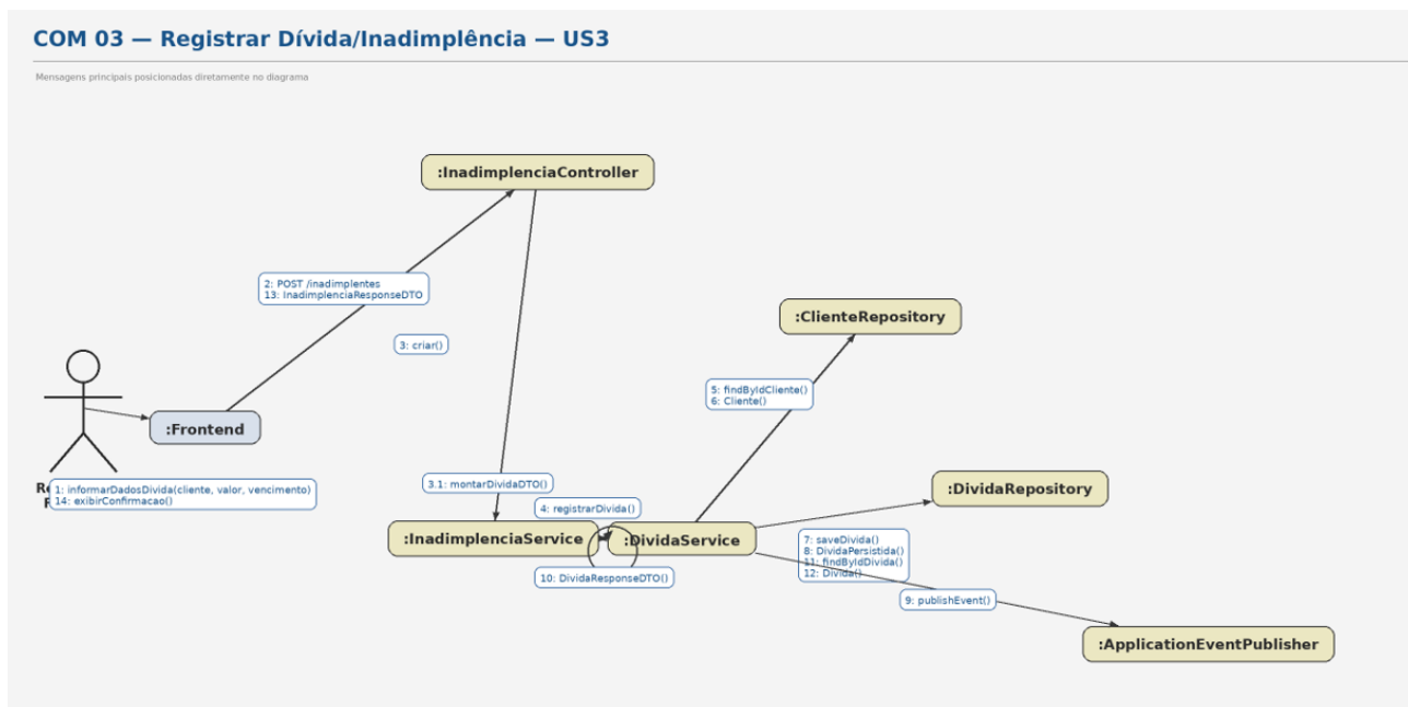
Figura 22 — Diagrama de Comunicação: Registrar Dívida.
