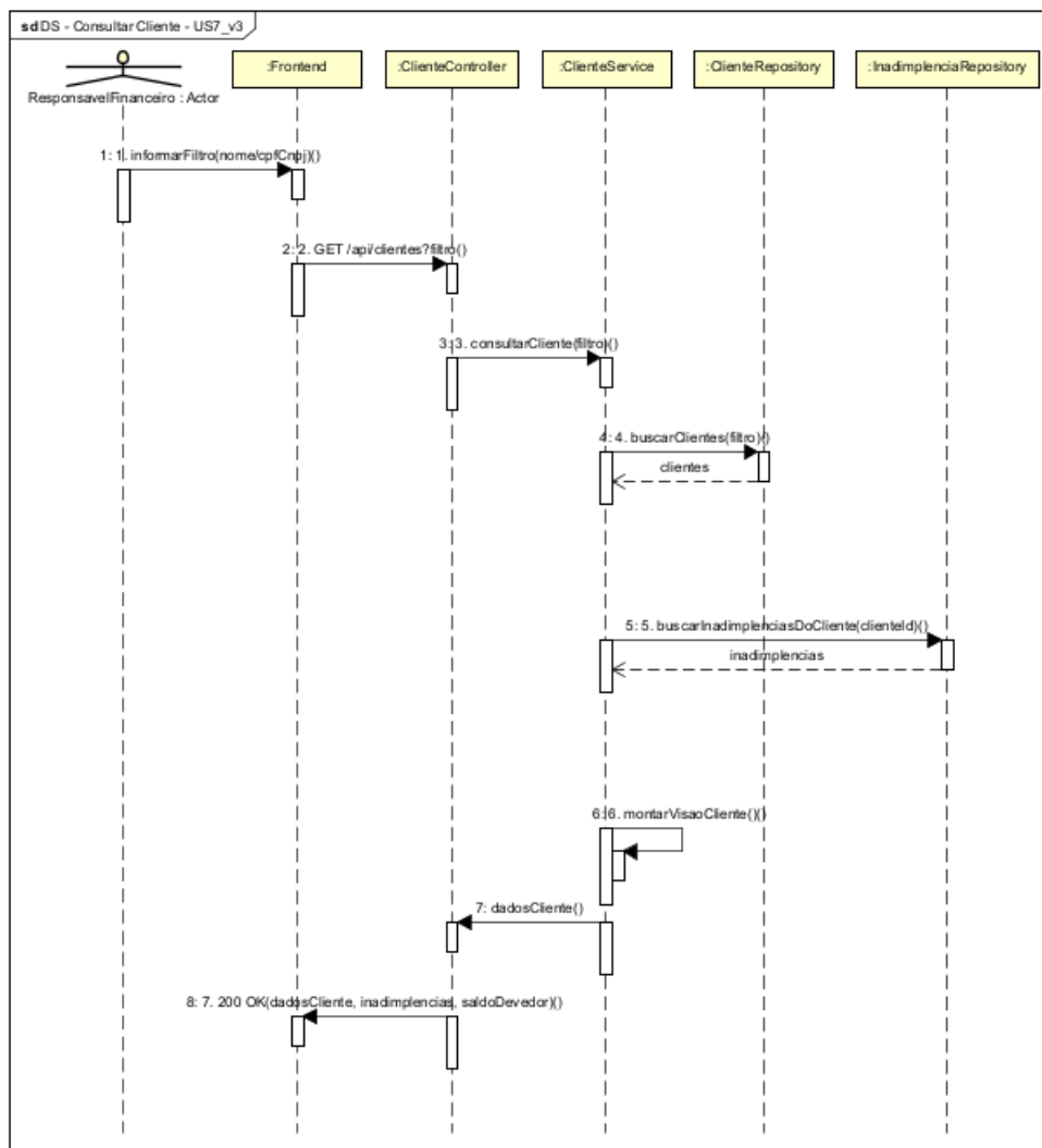
Figura 10 — Diagrama de Sequência: Consultar Cliente — US7.
