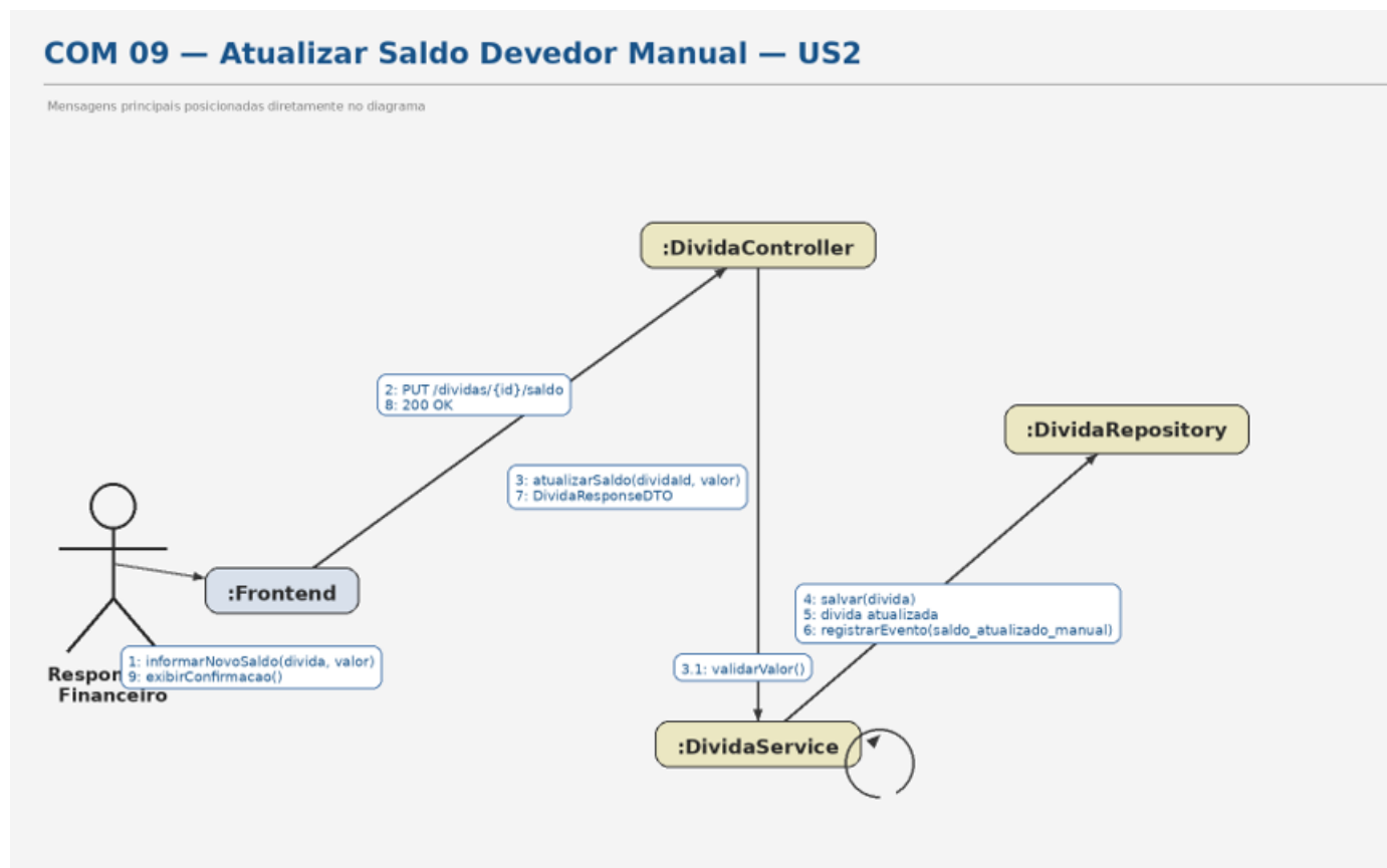
Figura 28 — Diagrama de Comunicação: Atualizar Saldo Devedor.
