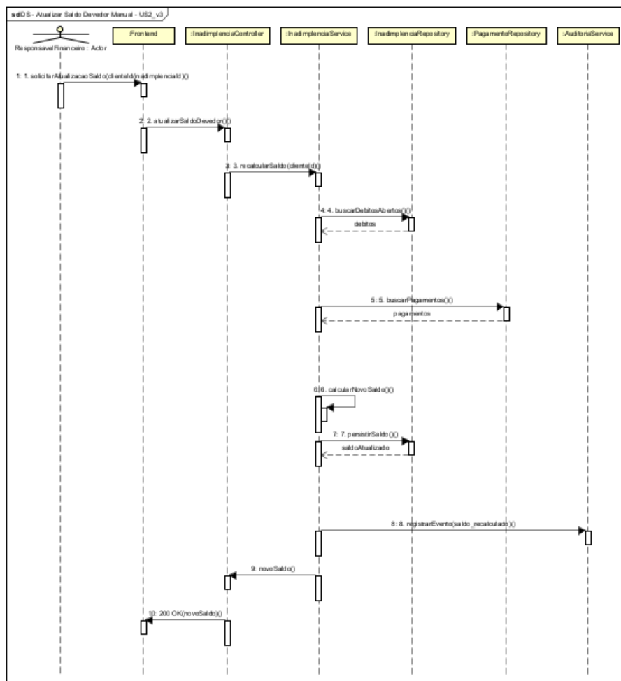
Figura 13 — Diagrama de Sequência: Atualizar Saldo Devedor Manual — US2.
