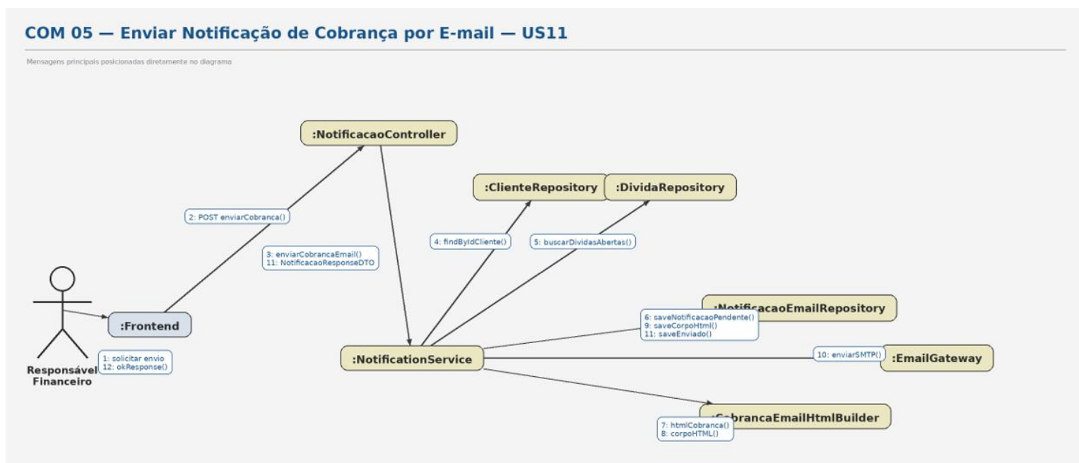
Figura 24 — Diagrama de Comunicação: Enviar Notificação de Cobrança por E-mail.
