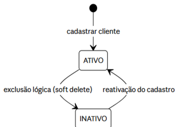
Figura 35 — Diagrama de Estado.
