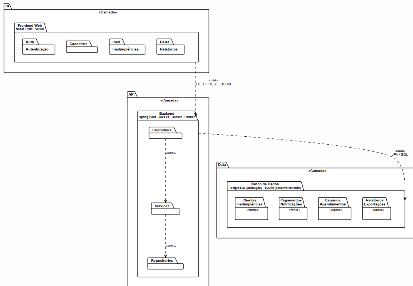
Figura 31 — Diagrama de pacote
