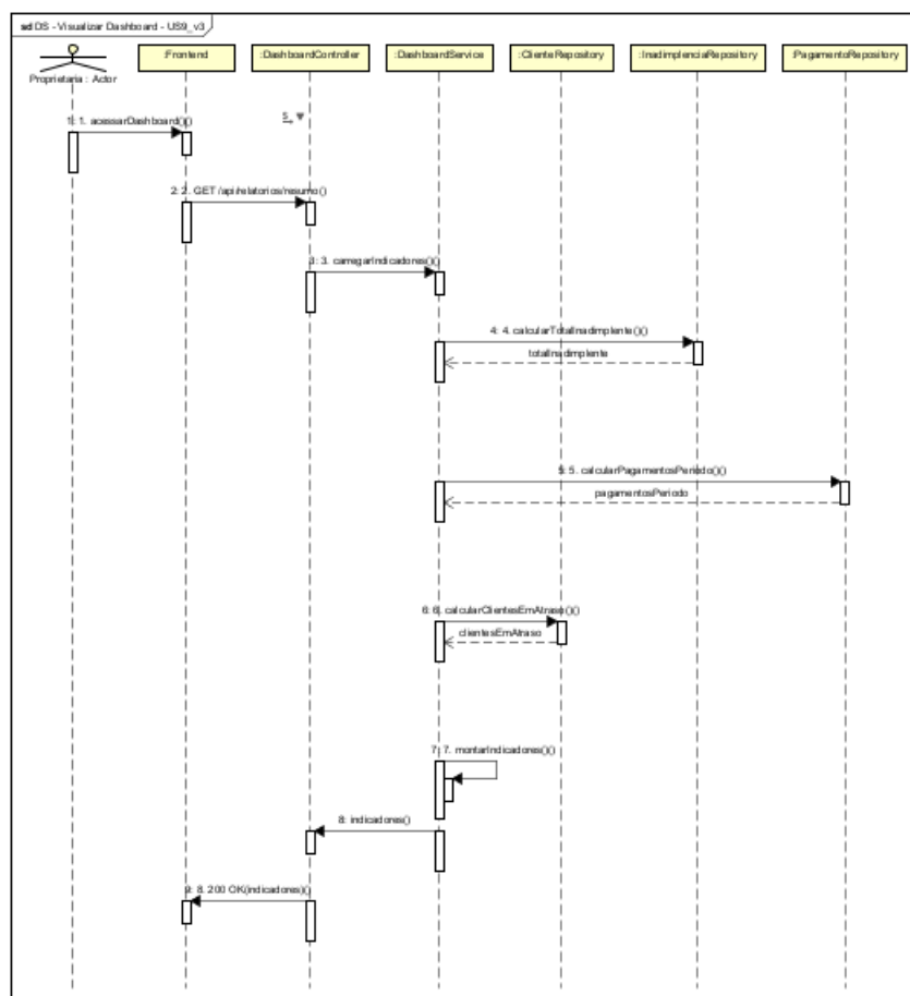
Figura 17 — Diagrama de Sequência: Visualizar Dashboard — US9.
