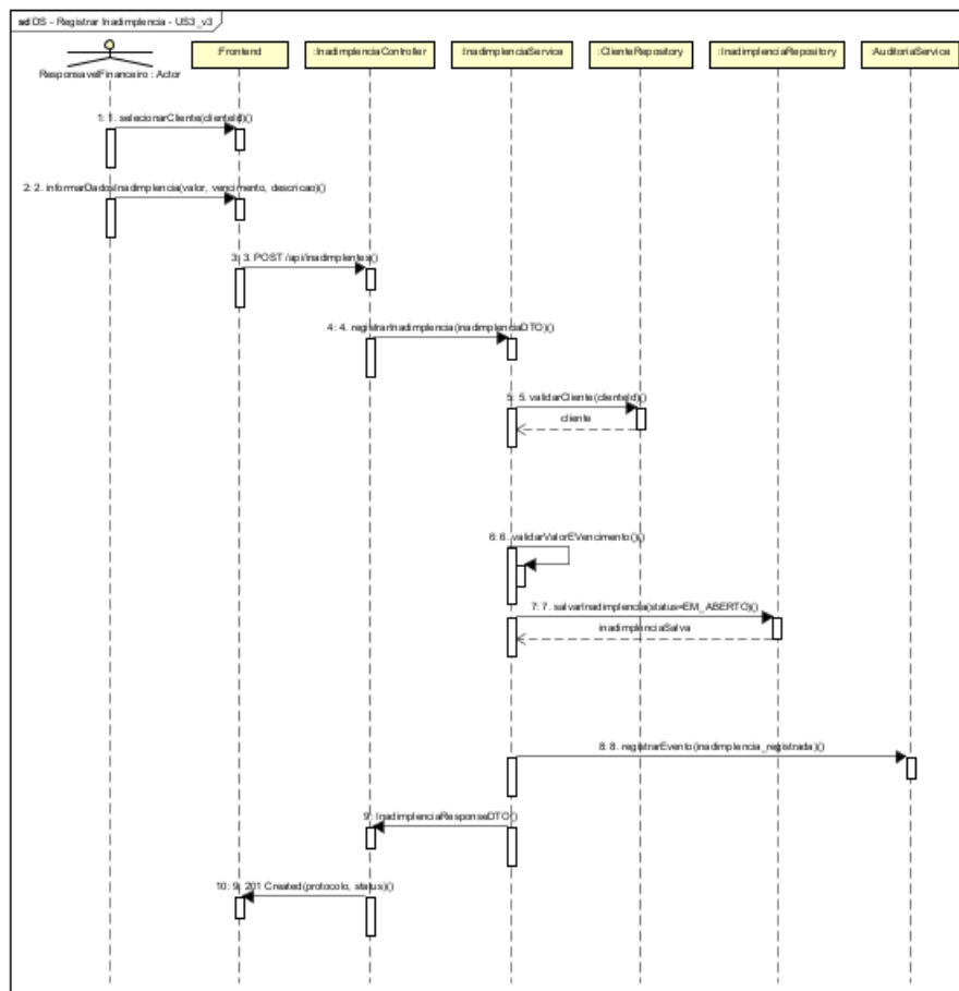
Figura 11 — Diagrama de Sequência: Registrar Inadimplência — US3.
