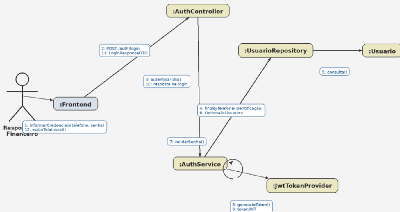
Figura 20 — Diagrama de Comunicação: Autenticar Usuário.
