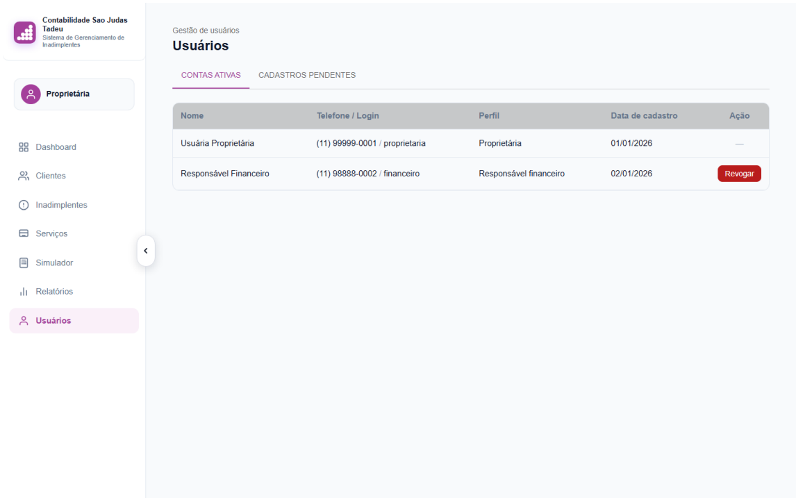
Figura 50 — Tela de Revogação de Acessos.
