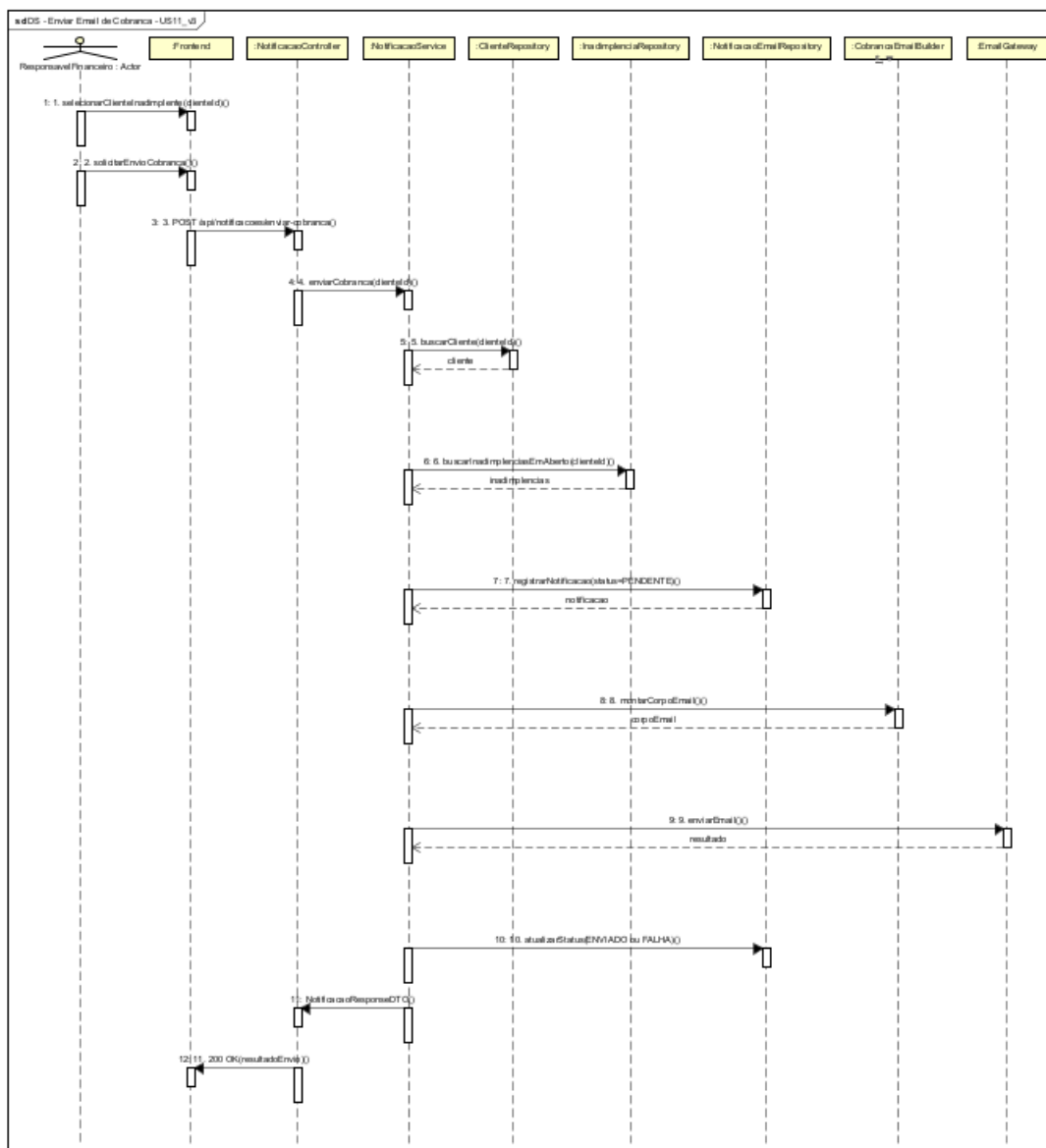
Figura 18 — Diagrama de Sequência: Enviar E-mail de Cobrança — US11.
