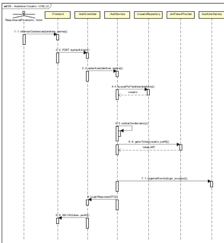
Figura 8 — Diagrama de Sequência: Autenticar Usuário — US8.
